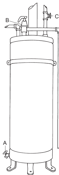
A: Válvula de drenaje B: Válvula de descarga de presión C: Válvula de Agua Fría
